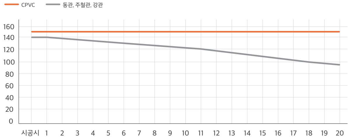
연수별 유체흐름계수(C)
